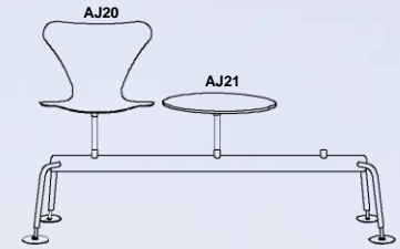
EV3L estrutura 3 lugares/ beam, 3 seats/ structure 3 assises L. 1550 P.480 A.800
